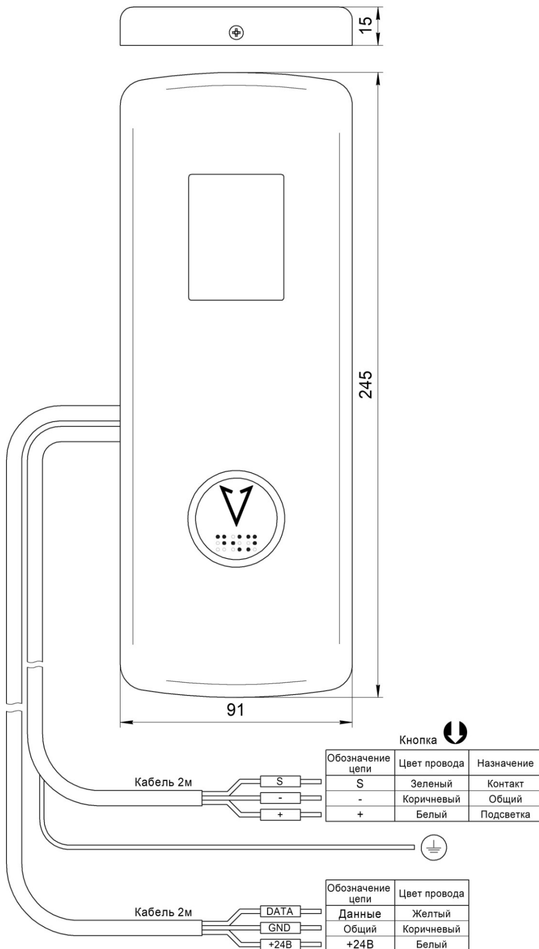
Рис.1 Внешний вид, габаритные и установочные размеры Вызывного поста ЦИРКОН НШЕК.468381.078-01
